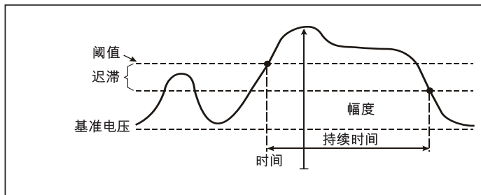
图示 7. 电压骤升的特征
