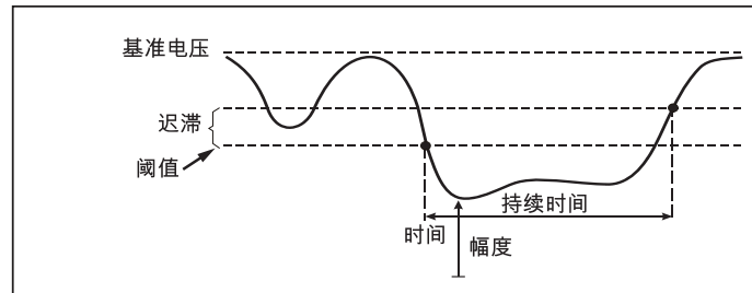
图示 8. 电压骤降的特征
