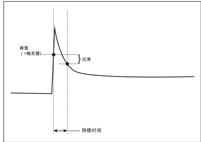
图示 10. 浪涌特征及与开始菜单的关系
