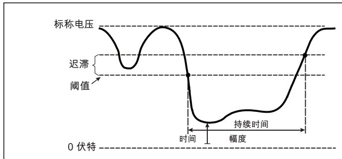
图示 9. 电压中断的特征
