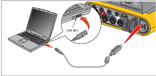
图示 12. Power Logger 至 PC 的连接
