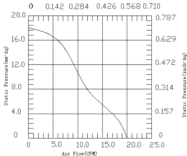
风扇风量风压特性图
