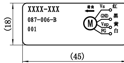
【铭牌二内容】
