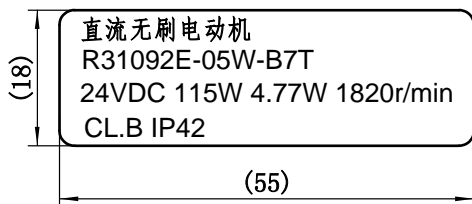
【铭牌一内容】
