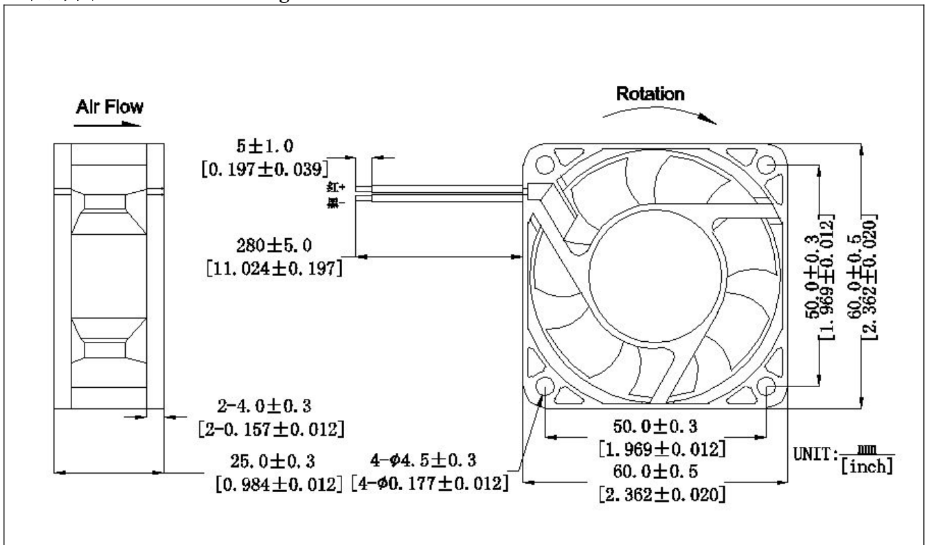
7. 尺寸图 Dimension Drawing
