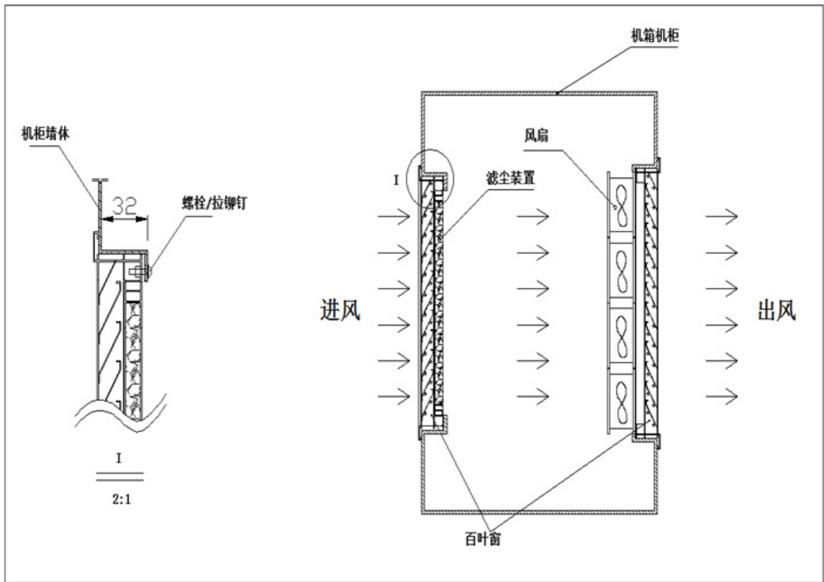
百叶窗与墙洞连接固定方案图 订购形式
