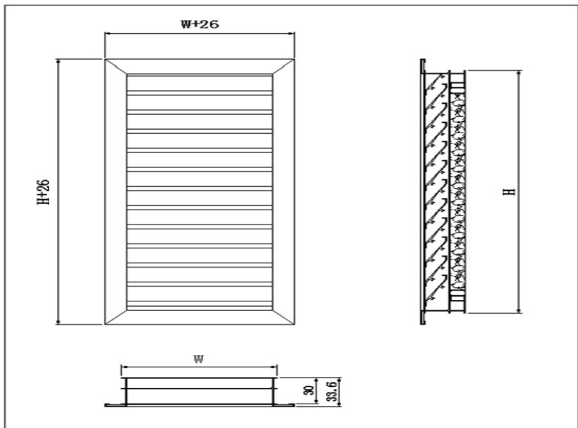
百叶窗与墙洞连接固定方案图 订购形式
