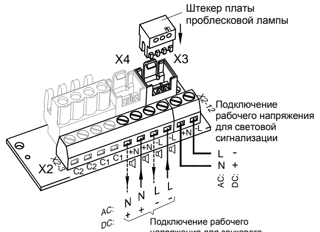
Раздельное подключение звукового и светового оповещения
