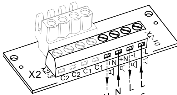
Подключения рабочего напряжения AC: N N L L DC: + + - -
