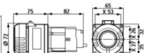
Flanschsteckdose/Flange socket/Prise à bride 2-pol./pôl. + PE
