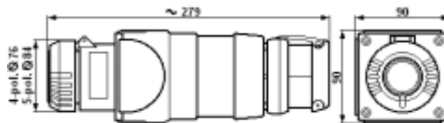
Kupplung / Coupler / Prolongateur 4/5-pol./pôl. + PE
