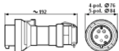
Stecker / Plug / Fiche GHG 511 4. 4/5-pol./pôl. + PE
