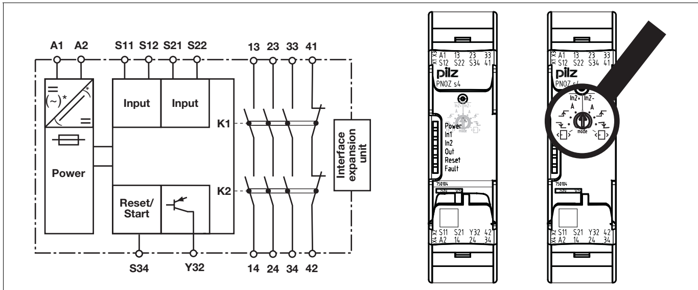
*nur bei U_B = 48 - 240 \text{ V AC/DC} Mitte: Frontansicht mit Abdeckung Rechts: Frontansicht ohne Abdeckung
