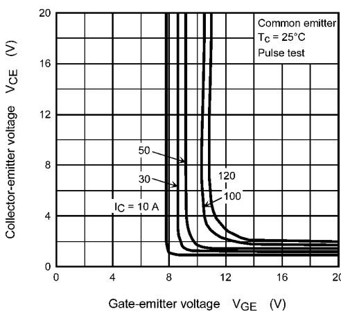
Fig. 8.5 V_{ce} - V_{ge}
