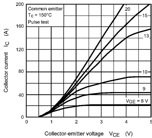
Fig. 8.4 I_c - V_{ce}
