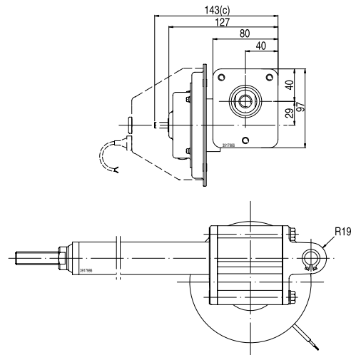
DC motor
