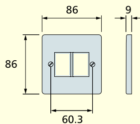
2 module K172 ALM
