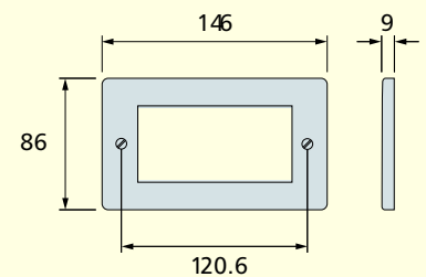
4 module K184 ALM
