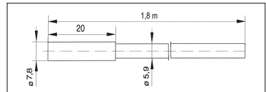
Afmetingen van de sensor
