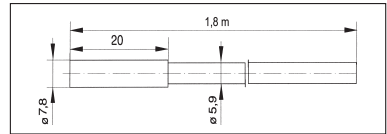
Temperaturgivarens mått
